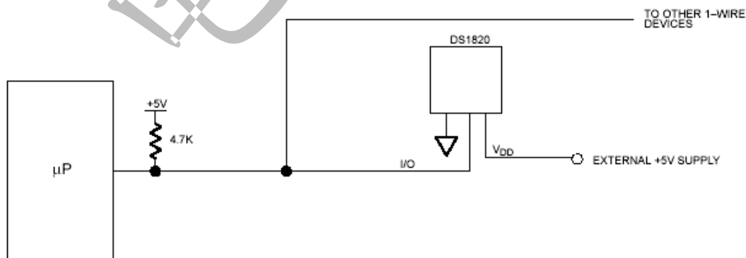
图 3 使用 V DD 供温度变换所需电流
